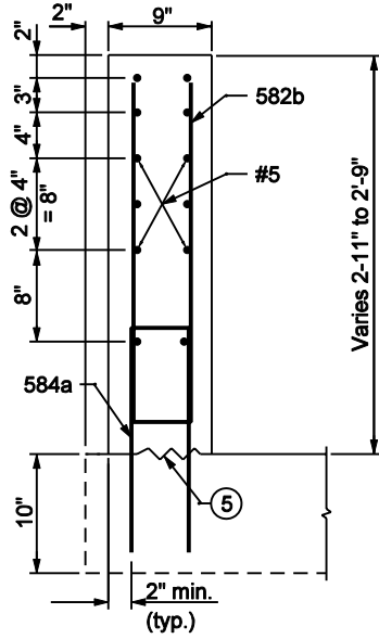
SECTION D-D
