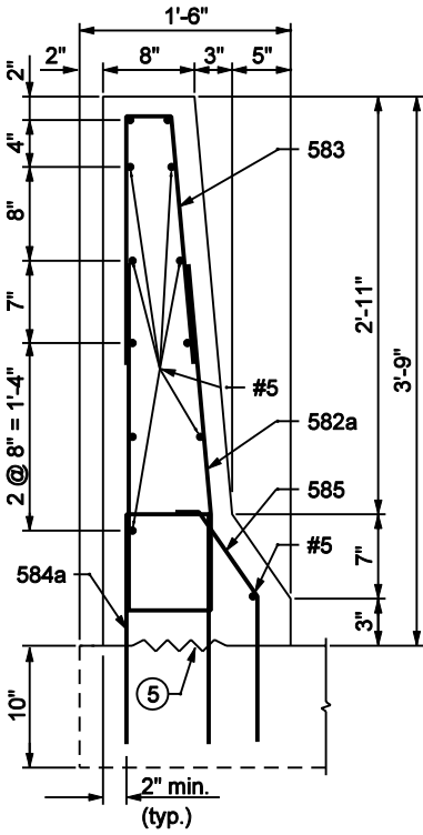
SECTION A-A
