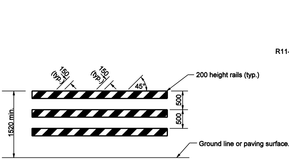
TYPE III BARRICADE
